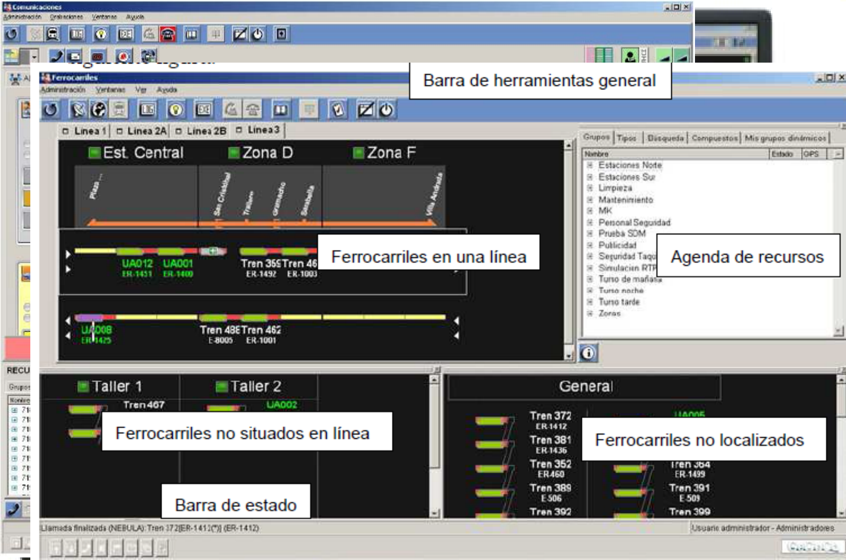
Figura 16: descripción de las partes del sinóptico de línea
